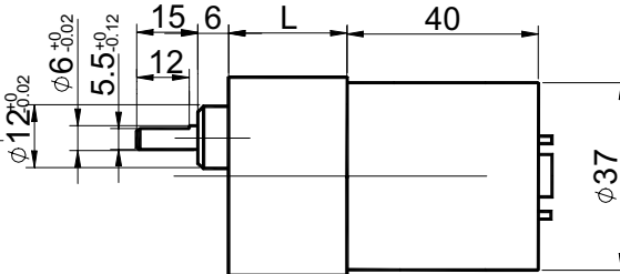
单扁平出轴
